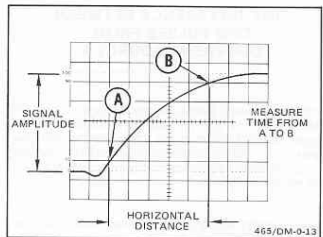
Fig. 19. Risetime.
