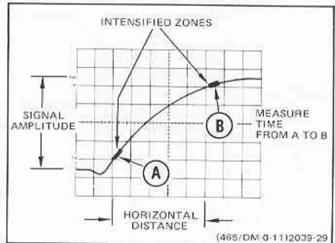
Fig. 32. Risetime.
