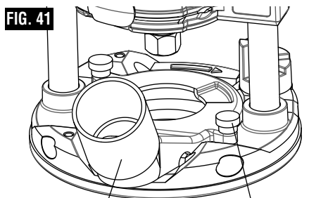
FIG. 41 CAPUCHON D'EXTRACTION DE POUSSIÈRE (accessoires en option)
